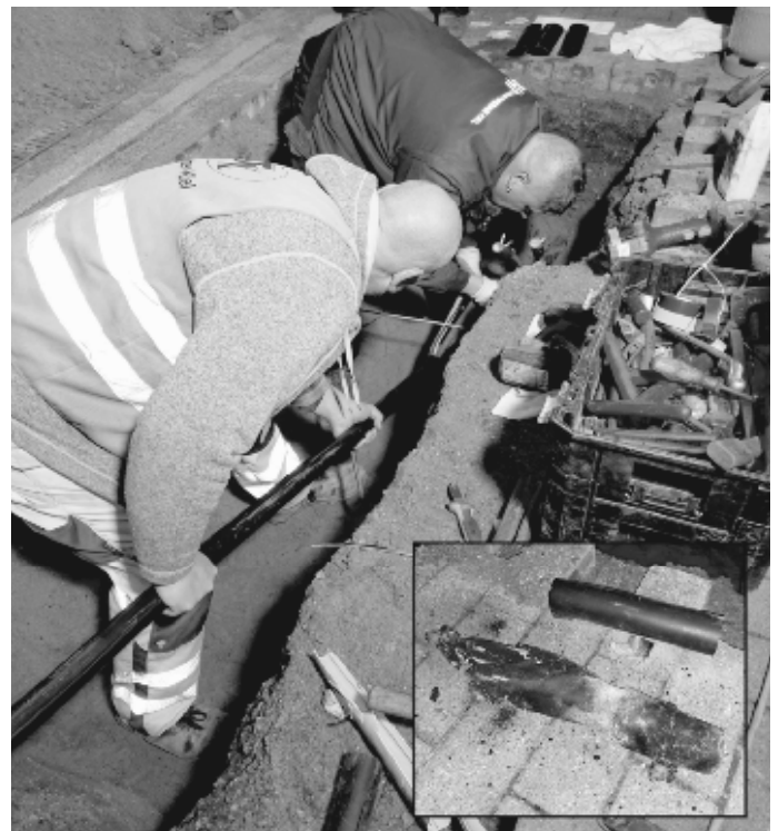
Notdienstmonteure setzen ein neues Erdkabel ein. Im Kasten ist die verbrannte Schadstelle zu erkennen.
